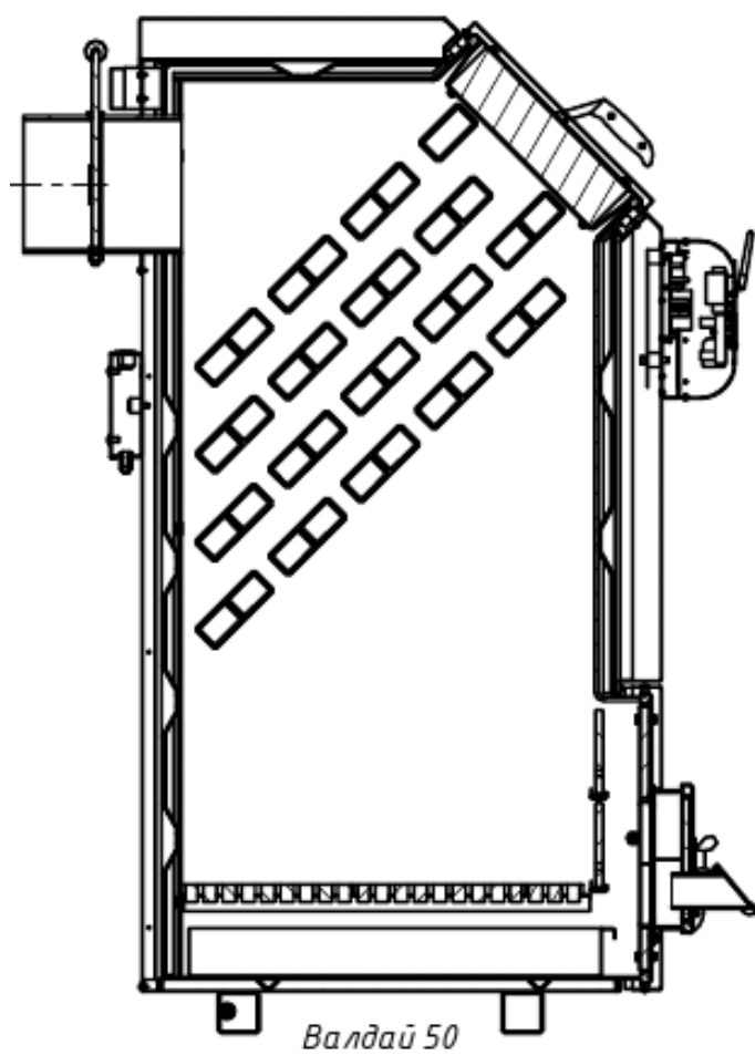
Рис. 1а. расположение заслонок в котлах Валдай.
