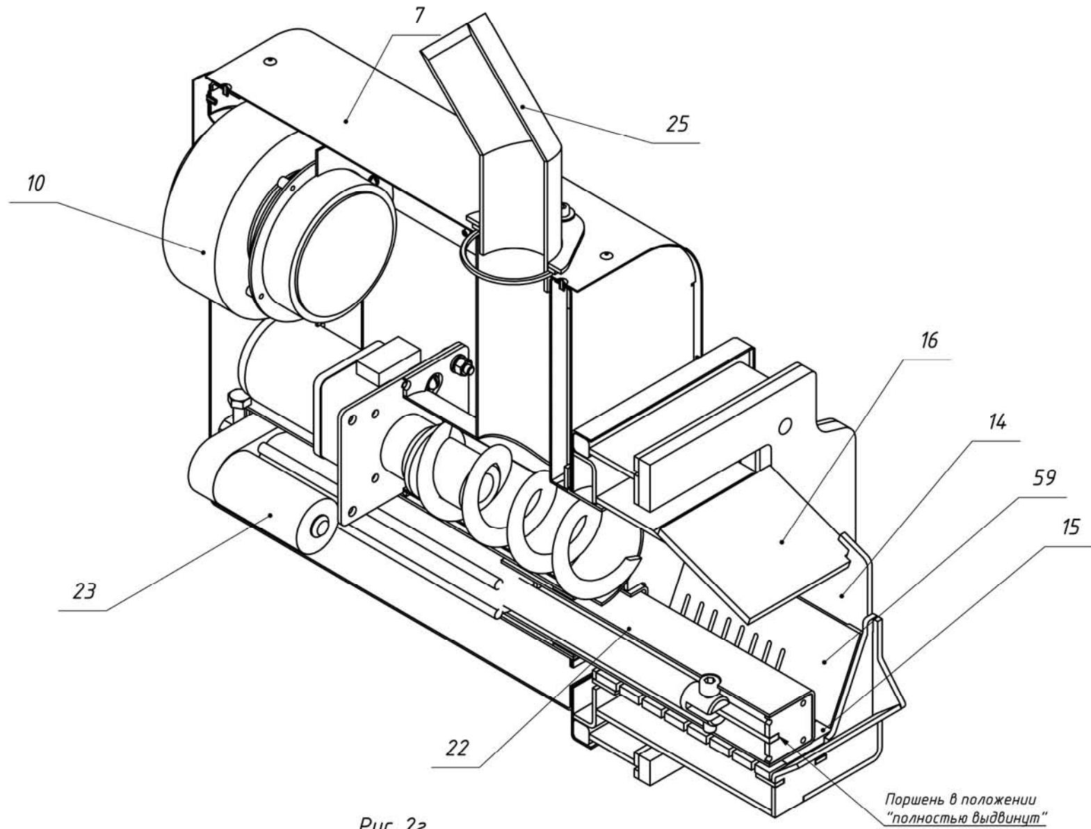
Рис. 22 Горелка пеллетная ВС 4/35Е (ВС 10/50Е).
