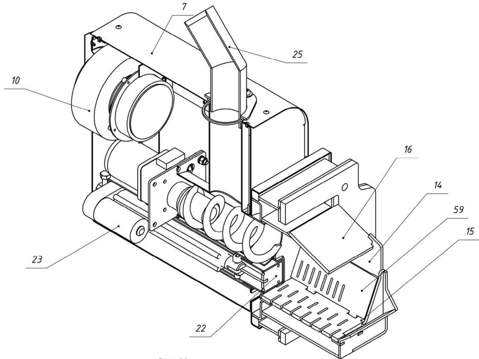
Рис. 28 Горелка pelletная BC 4/35E (BC 10/50E).
